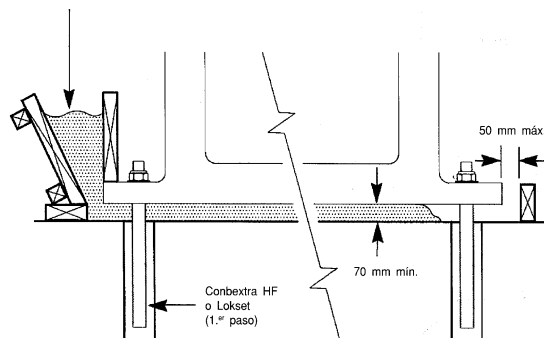
Figura 1: Cimentación habitual Vertido de Conbextra GV (2.º paso)
